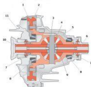
Схема дифференциала
